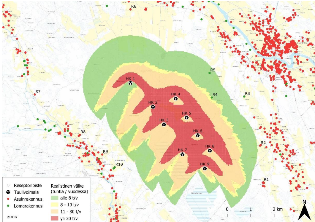
Kuva 3-2. Välikkeen realistinen määrä tunteina vuodessa (auringonpaistehavainnot otettu huomioon) Hangaskurunkankaan yhdeksän voimalan sijoitus suunnitelmalla. Mallinnus on tehty tuulivoimaloilla, joiden napakorkeus on 200 m ja roottorin halkaisija 200 m.
