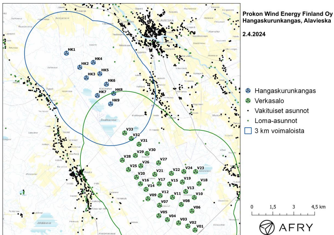
Kuva 5-1. Hangaskurunkankaan ja Verkasalon tuulivoimalat. Karttaan on piirretty vyöhykkeet 3 km etäisyydelle voimaloista.
