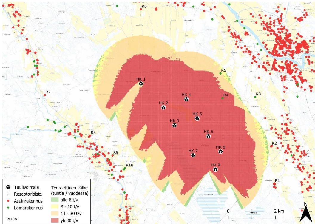
Kuva 3-1. Välikeen teoreettinen määrä tunteina vuodessa (auringonpaistehavaintoja ei ole huomioitu) Hangaskurunkankaan yhdeksän voimalan sijoitussuunnitelmalla. Mallinnus on tehty tuulivoimaloilla, joiden napakorkeus on 200 m ja roottorin halkaisija 200 m.
