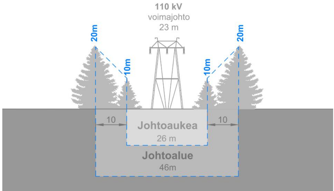
Kuva 134. Johtoalueen yleiskuvaus 110 kV voimajohtotyypillä. (A-Insinöörit Suunnittelu Oy).
