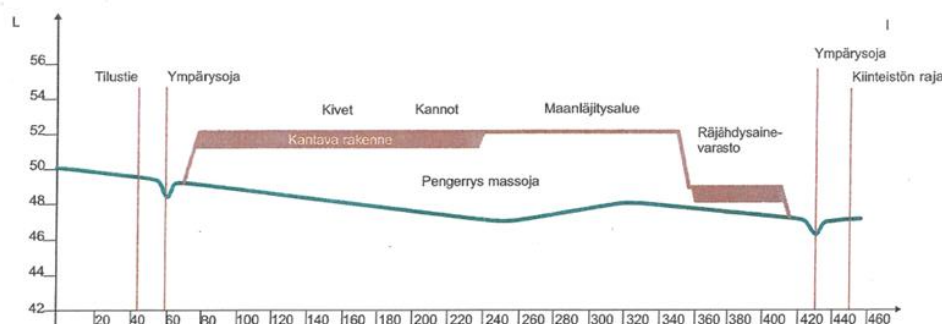
Kuva 3. Varasto- ja läjitysalueen pituusleikkaus.
